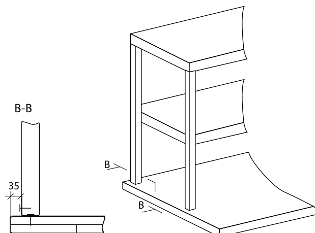
DM-P-3139 Nadstawka na stół
