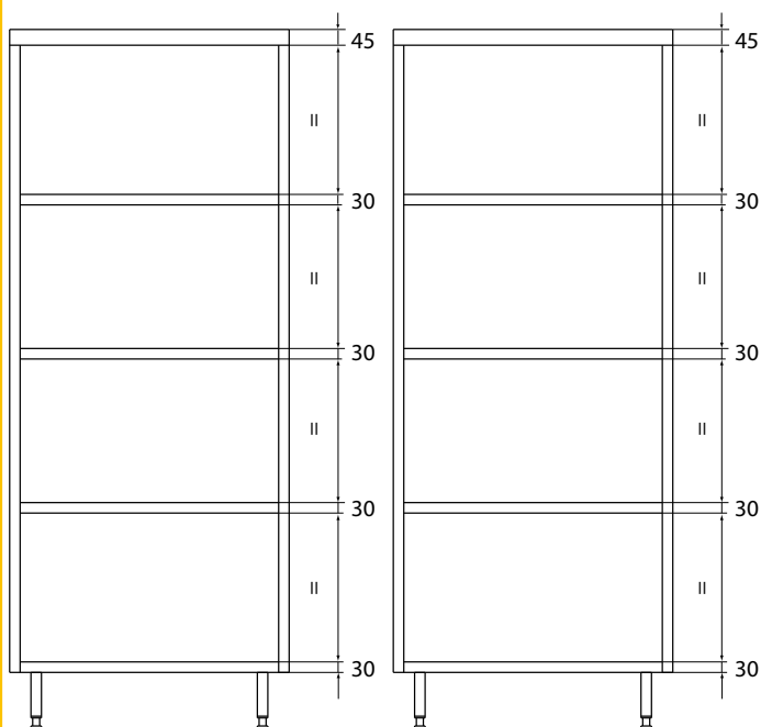
DM-P-3305.02 DM-P-3333.02 DM-P-3334.02
